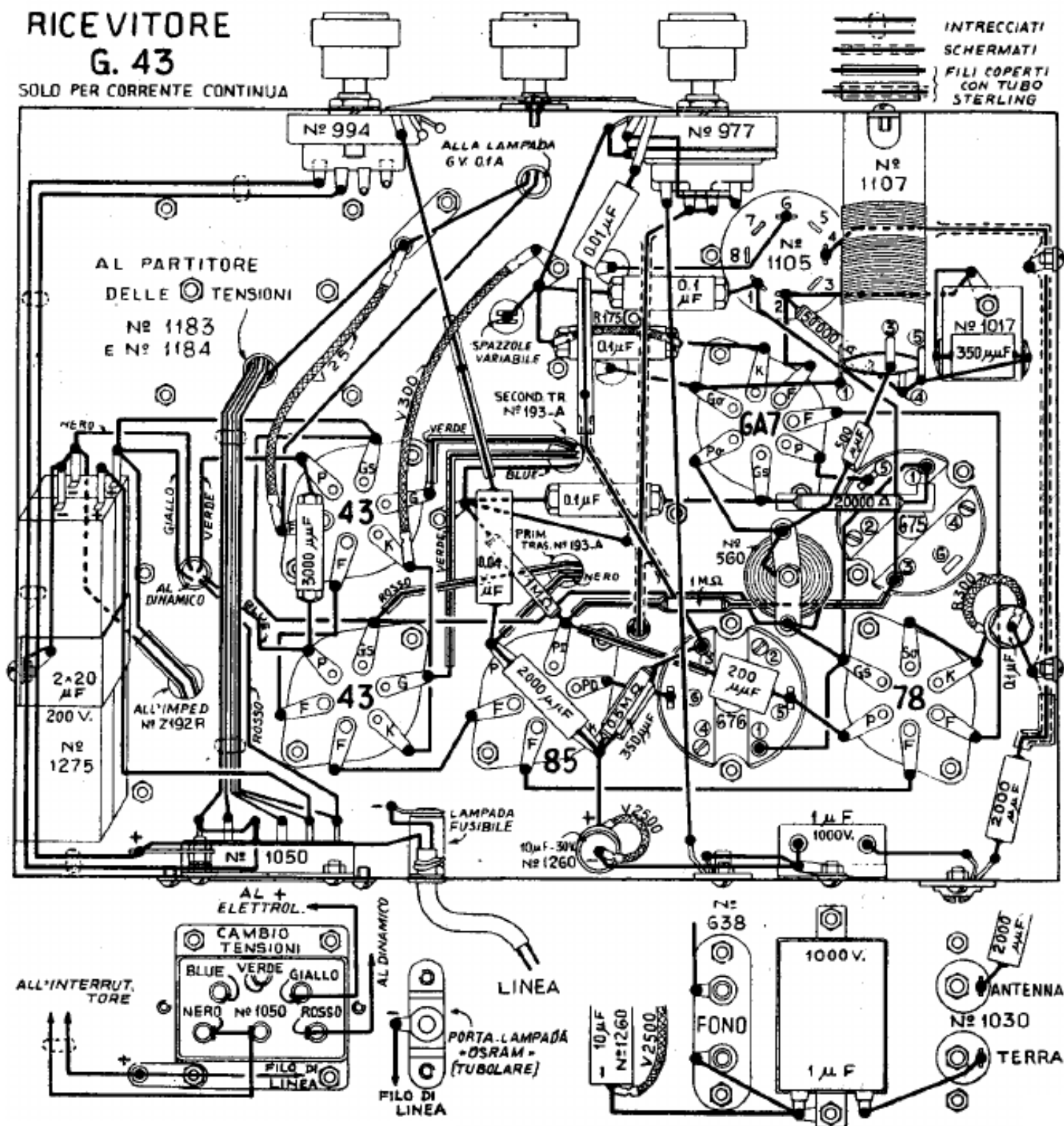
Piano di costruzione.
